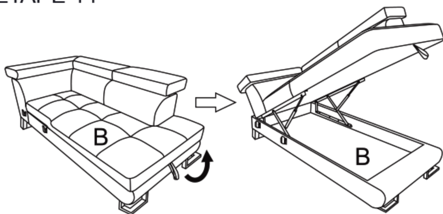
ÉTAPE 11
